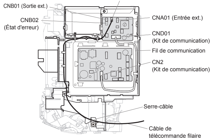
CNC01 (Télécommande filaire)
